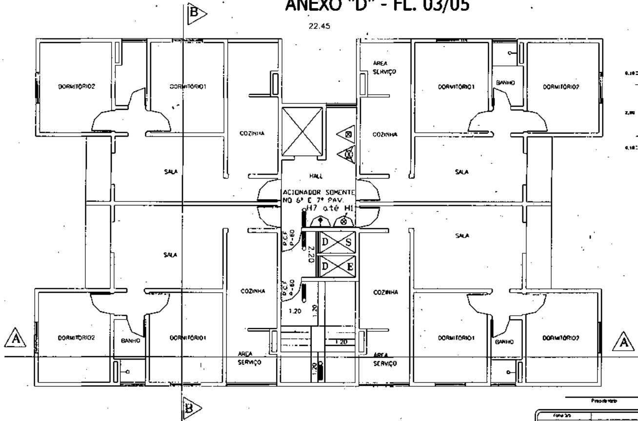
ANDAR TIPO - 1º AO 9º PAVIMENTO
