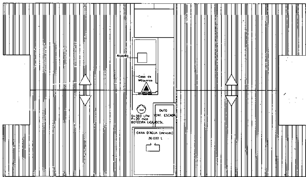
PLANTA DE COBERTURA - BLOCO 1 e 2
