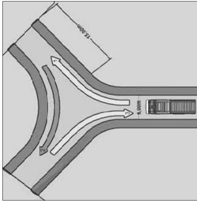
Figura 2: Retorno em formato de "Y"
