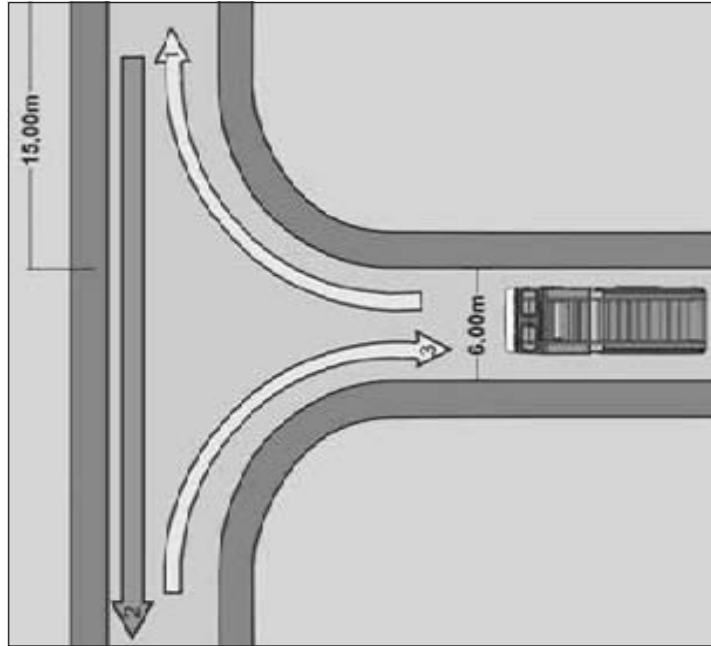
Figura 3: Retorno em formato de "T"
